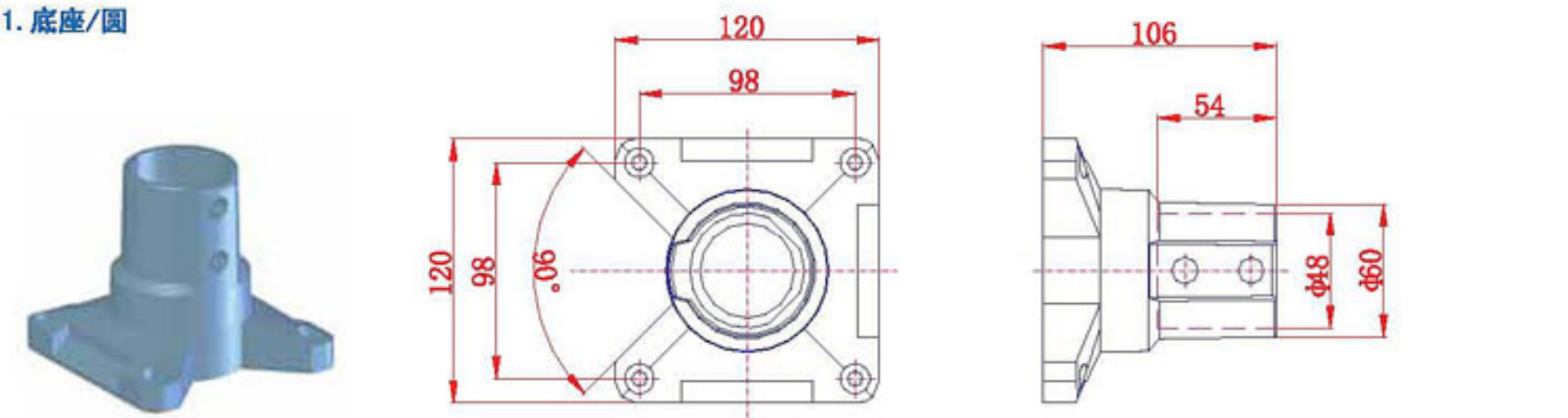
11. 底座/圆
